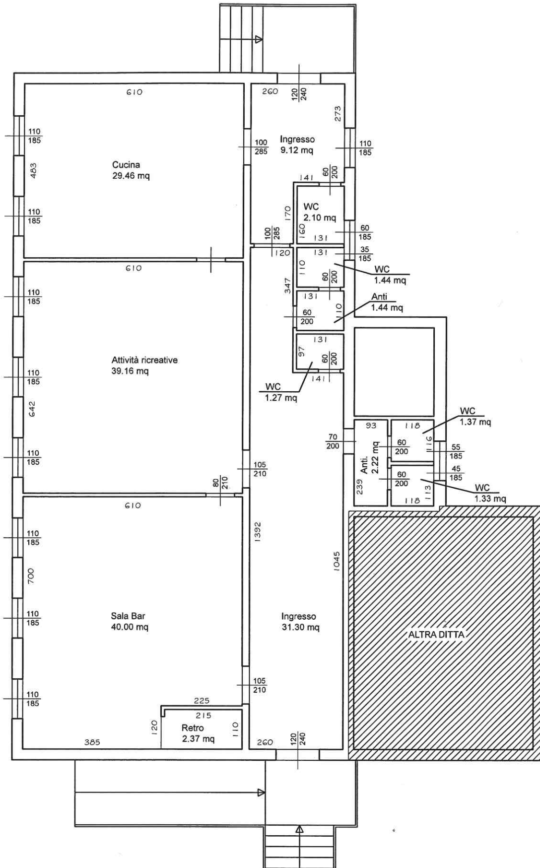
STATO DI FATTO PIANO TERRA H = 3.00 m
